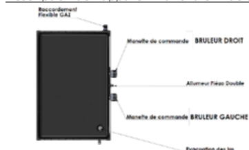
Description de l'appareil Plancha en vue dessus
