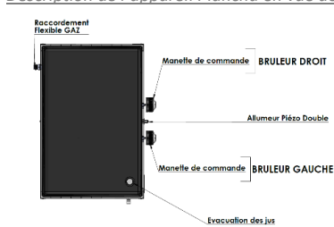
Description de l'appareil Plancha en vue dessus
