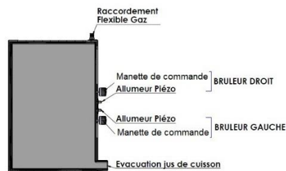
Description de l'appareil Plancha en vue dessus
